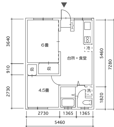
4.5畳+6畳+台所・食堂タイプ 12坪(40㎡)
